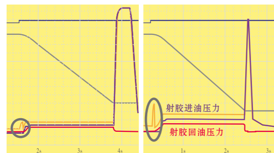
SPEED 168 平顺、无超调 竞争品牌160吨 压力不稳定、超调严重
