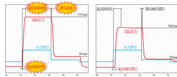
SPEED 168 动作响应快控制准确 竞争品牌160吨 动作响应慢，压力控制差
