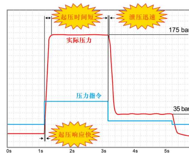
JM168-MK6 两段保压压力波形
